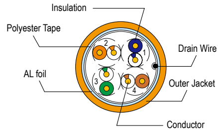
Cross section P/N: CLA04-SC5E
